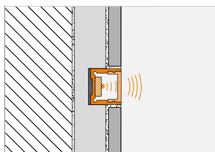
Osvětlený pás na 19 mm Schlüter-KERDI-BOARD-K
